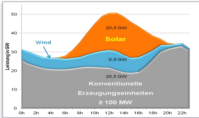
Wachsender PV-Strom-Anteil im Netz (hier EEX-Werte am 16.06.2013)
